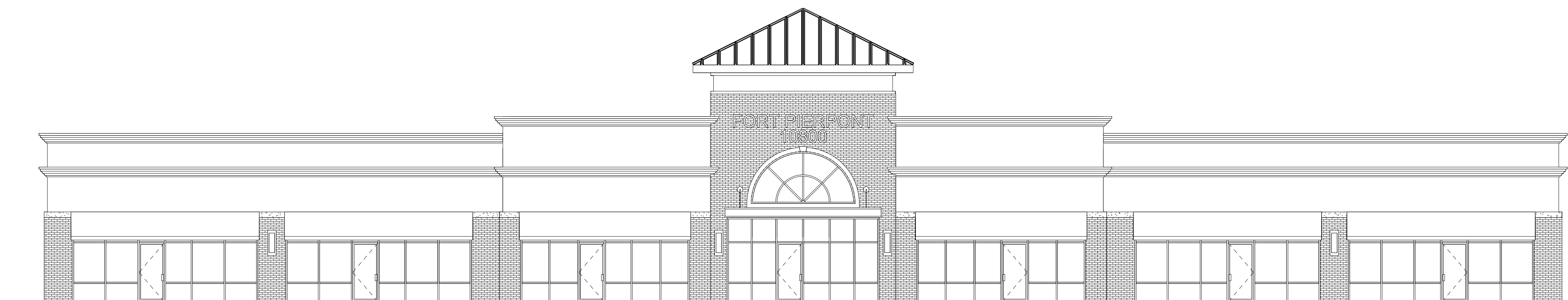
MAIN ELEVATION SCALE: 1/8" = 1'-0"
